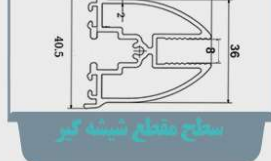
سختاب مقطع نشسته گیر
