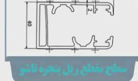
سختاب مقطع ریل پنجره تاشو
